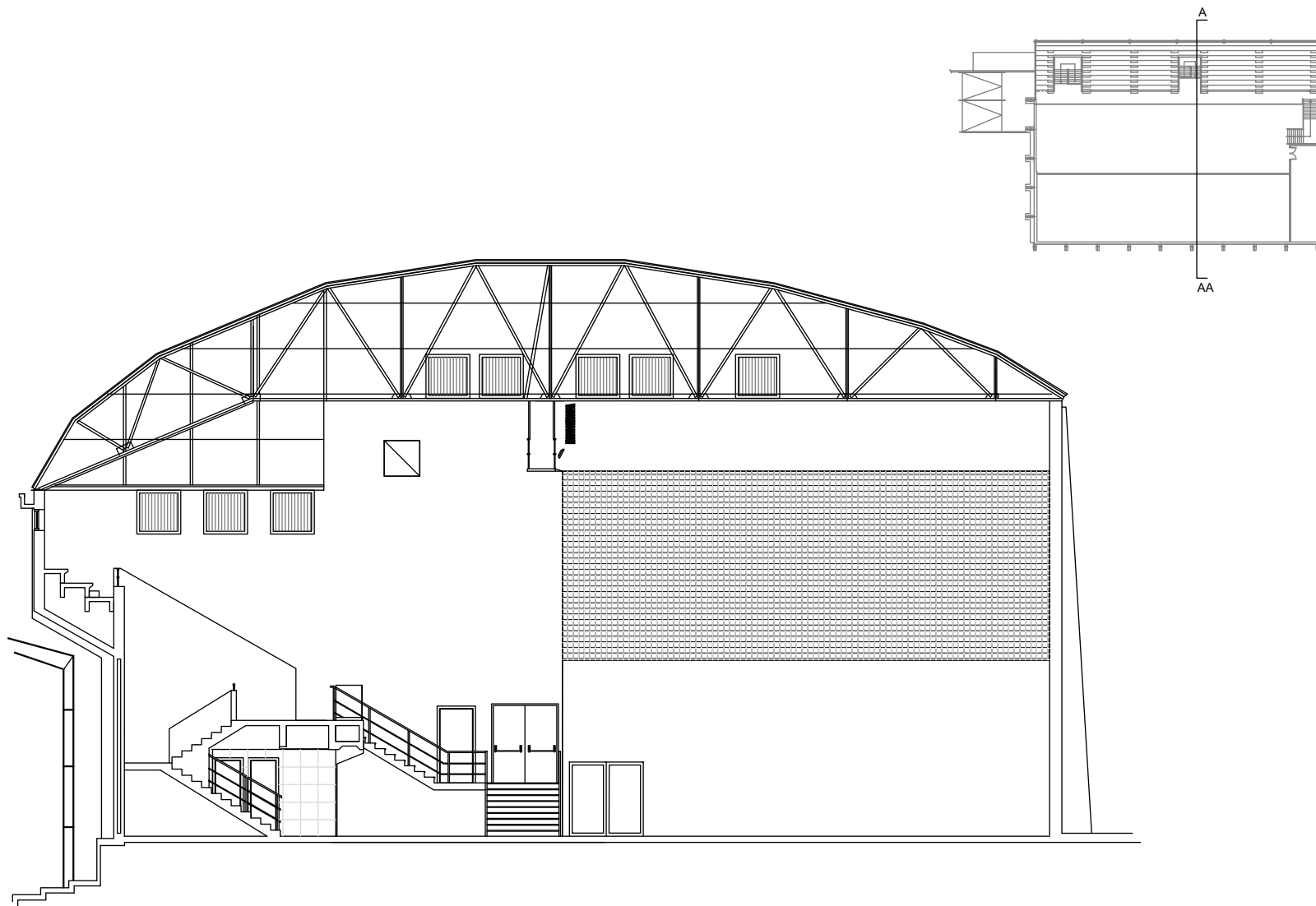
SECCIÓN A- AA
