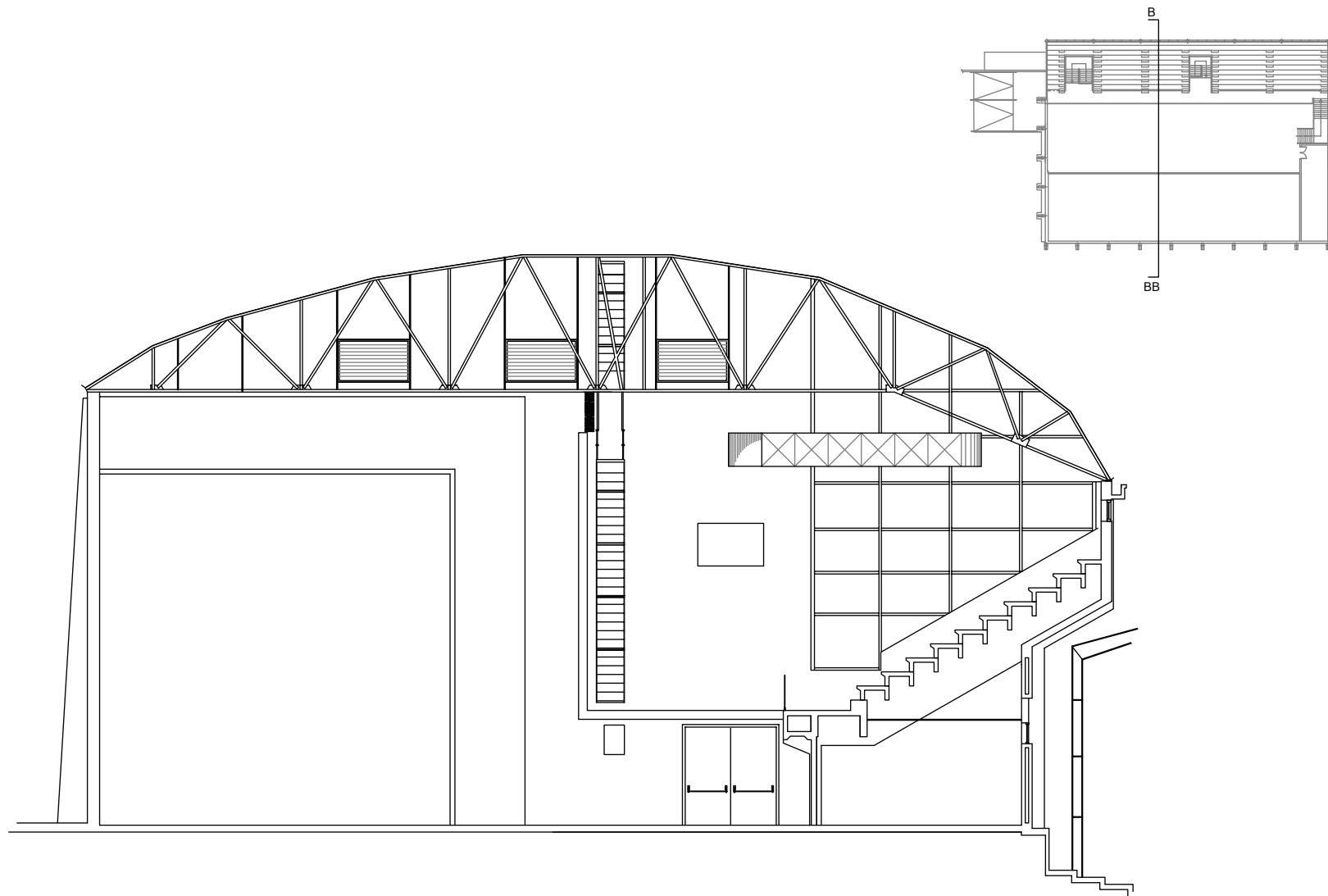
SECCIÓN B - BB
