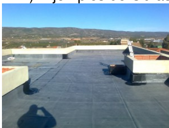
Continuidad en las Cubiertas con EPDM
